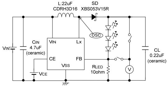
●Circuit ②
