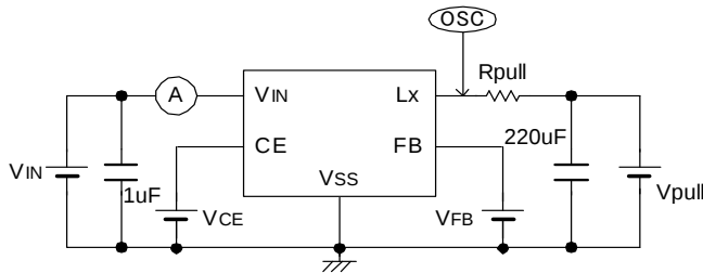
●Circuit ②
