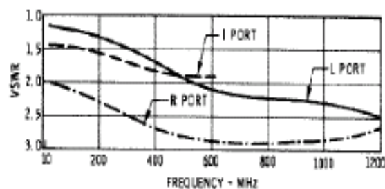
VSWR
