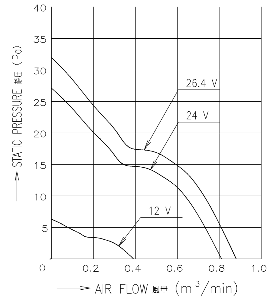
風量-静圧特性例
