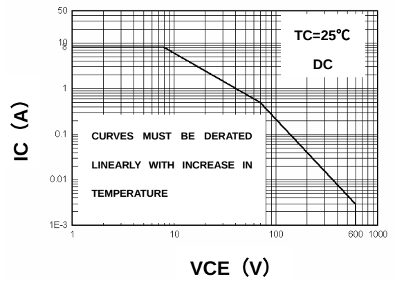
SOA
