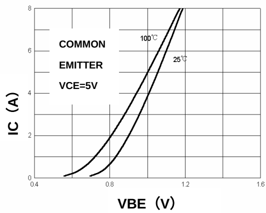
IC - VBE
