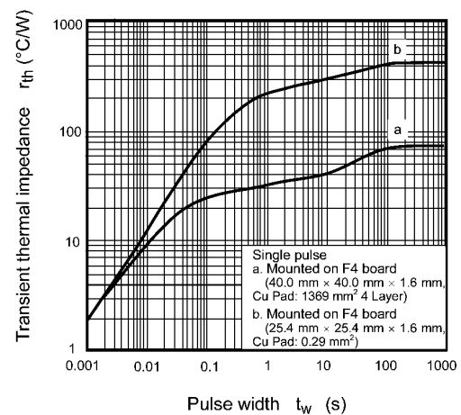
Fig. 7.12 r_{th} - t_w
