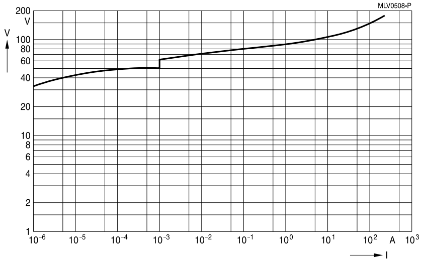
CT1206K35G
