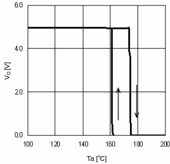
Fig. 28 TSD ( I_o=0\text{mA} )
