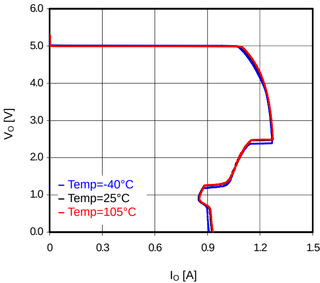
Fig. 29 OCP
