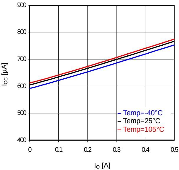
Fig. 30 I_O-I_{CC}
