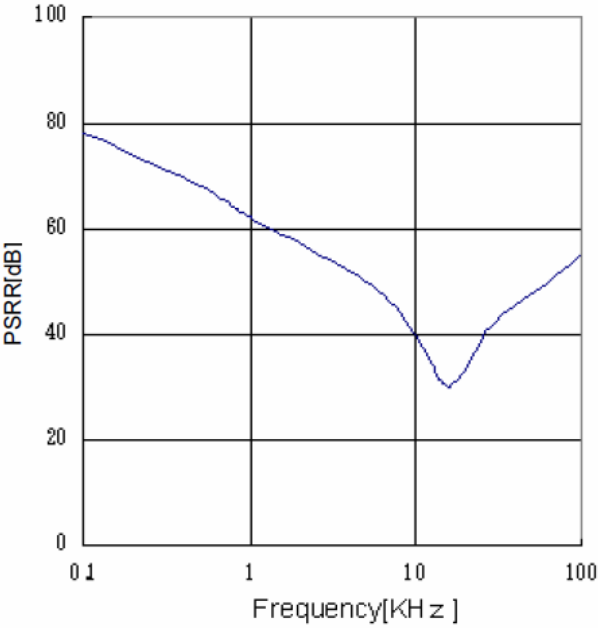
Fig. 32 PSRR ( I_o=0mA )
