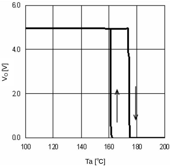
Fig. 28 TSD ( I_o=0mA )
