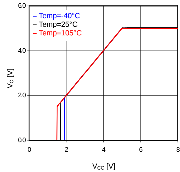
Fig. 27 V_{CC}-V_O ( I_O=0\text{mA} )
