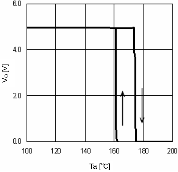
Fig. 28 TSD ( I_o=0mA )
