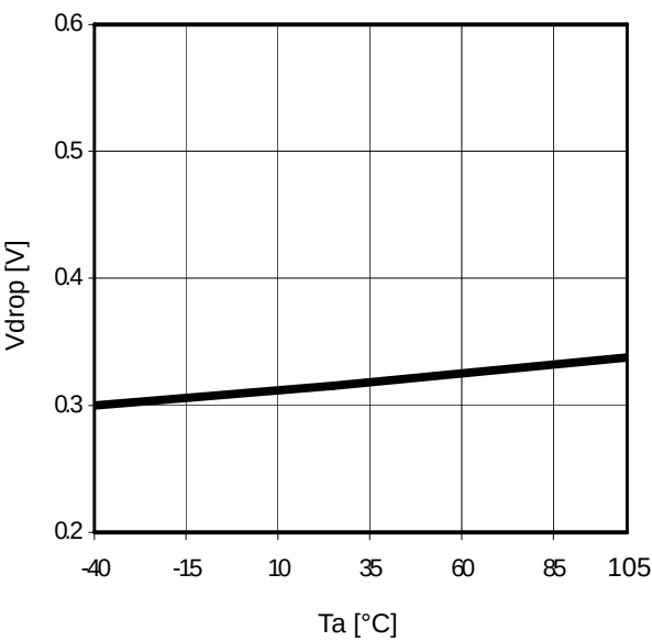
Fig. 33 Ta-Vdrop ( V_{CC}=6V , I_o=0.5A )
