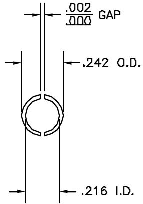
VIEW A-A
