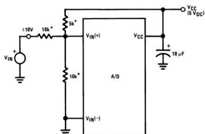
Figure 28. Handling \pm 10\text{V} Analog Inputs
