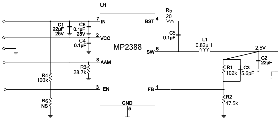
Figure 12: V_{IN} = 19V , V_o = 2.5V , I_o = 1A
