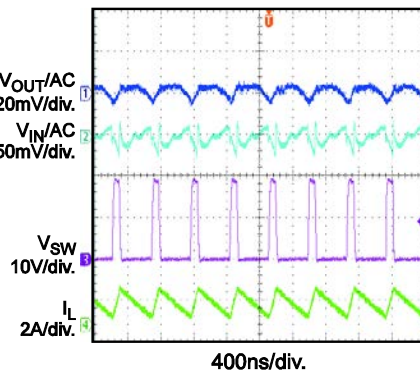
Input/Output Ripple
