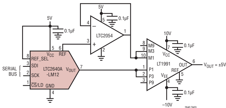
Programmable \pm 5\text{V} Output
