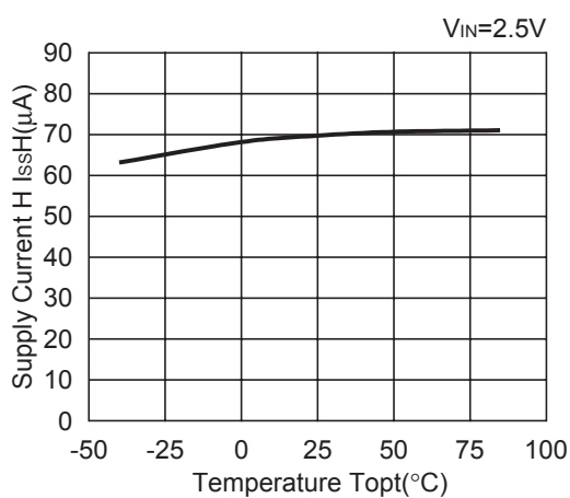
R1163x151x ECO=H
