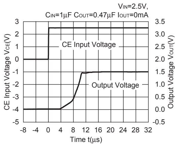
R1163x151x ECO=H
