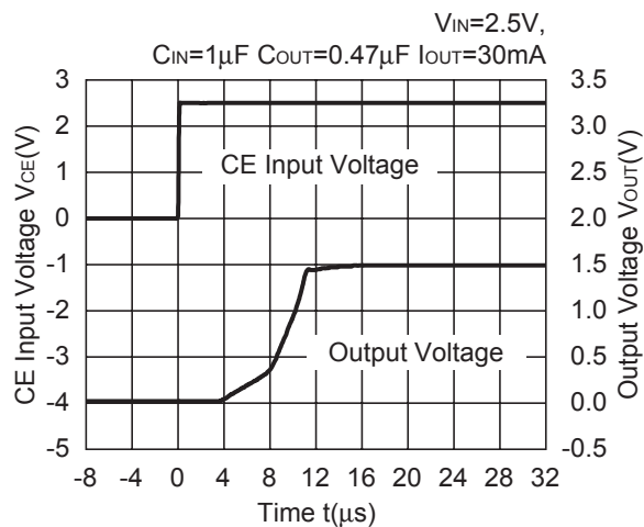
R1163x151x ECO=H
