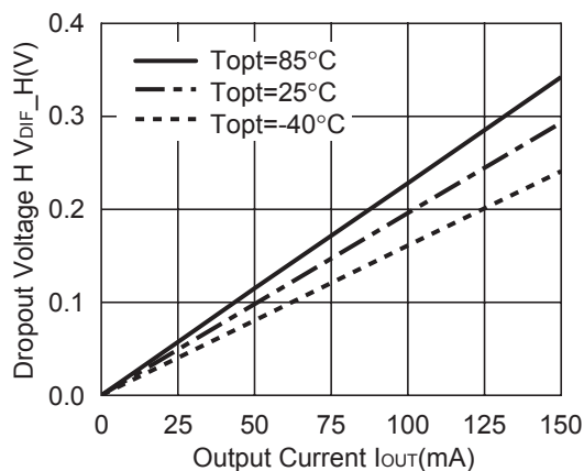
R1163x211x ECO=H
