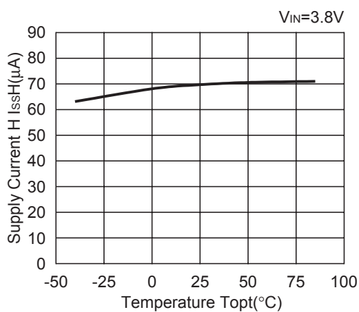
R1163x281x ECO=H
