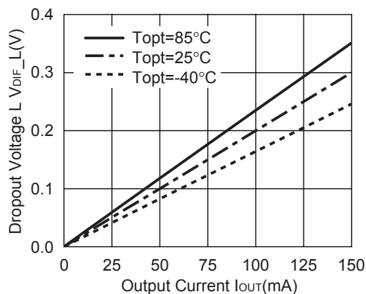
R1163x211x ECO=L
