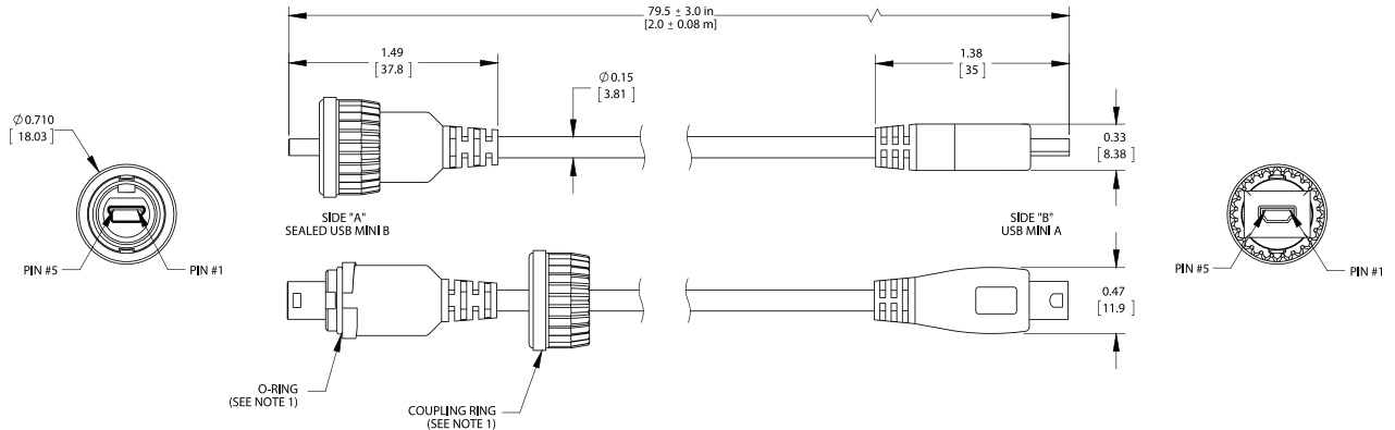
DCM-USBNB-USMAR2 Sealed USB 2.0 Mini B Plug to USB 2.0 Mini A Plug
