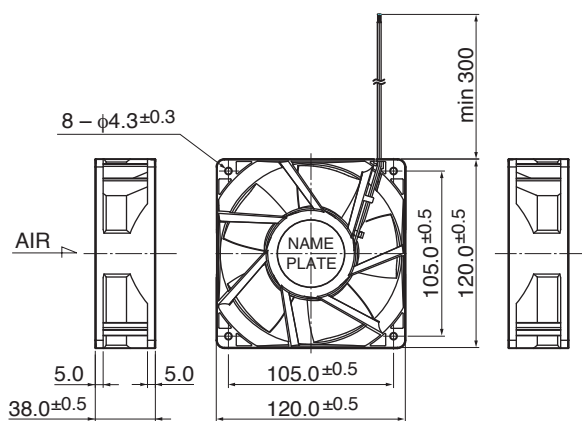
* 外観図は E (フランジ) タイプ Outline is E (Flange) type.
