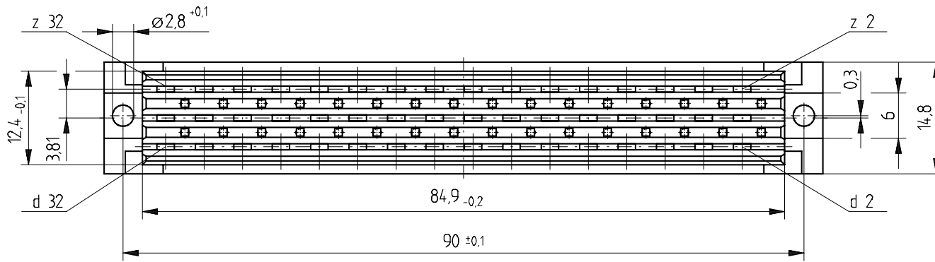
Bestückungsplan / contact layout
