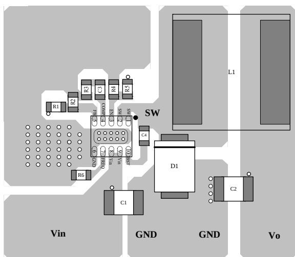
TOP Layer
