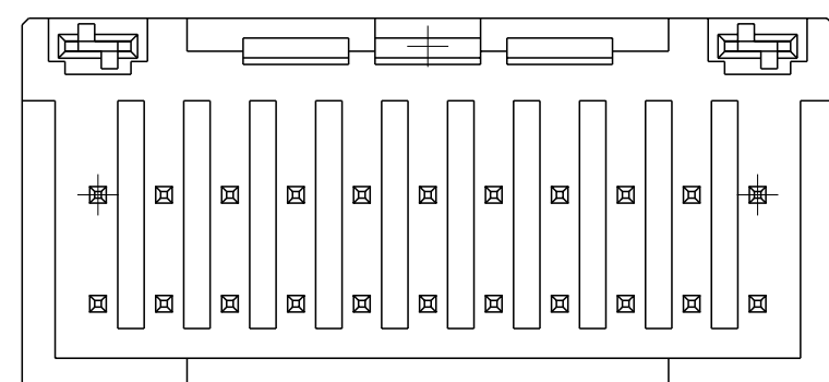
22POS(X-KEY): I-1827872-1
