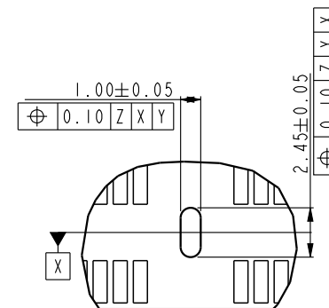
Center forklock type
