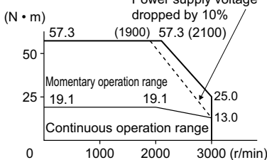
R88M-K4K020(H/T)-□ (4 kW)
