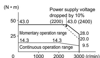
R88M-K3K020(H/T)-□ (3 kW)
