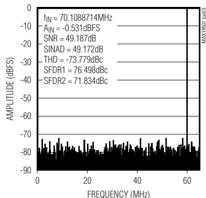
70MHz INPUT FFT PLOT
