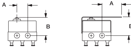
FIG. 1 Pin Plunger
