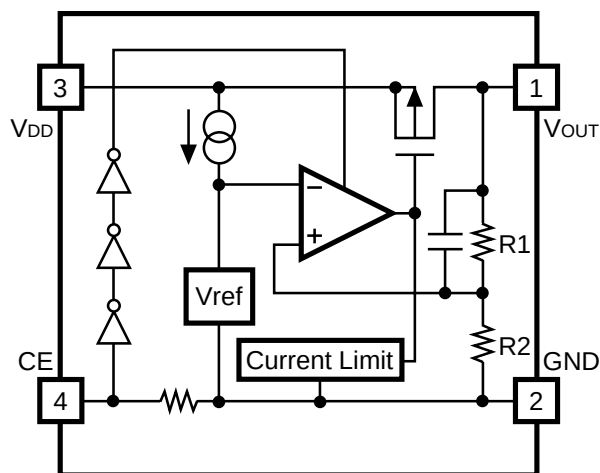
R1121NXX1B
