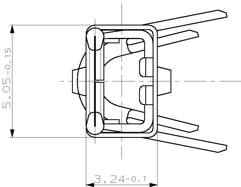
ANSICHT X
