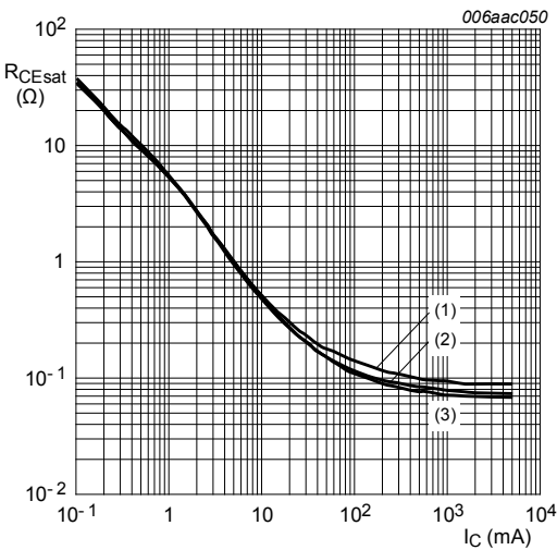
I_C/I_B = 20 (1) T_{amb} = 100^\circ C (2) T_{amb} = 25^\circ C (3) T_{amb} = -55^\circ C
