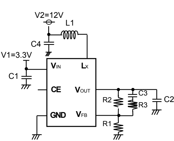
Fig 1. R1205x8xxA
