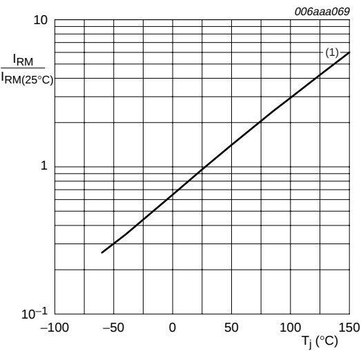
(1) PESD3V3L2BT, PESD5V0L2BT PESD12VL2BT, PESD15VL2BT and PESD24VL2BT: I_{RM} < 20\text{ nA} ; T_j = 150\text{ }^{\circ}C
