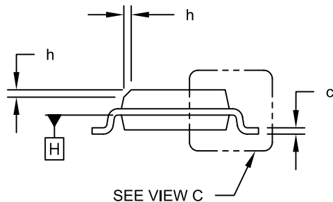
VIEW A-A
