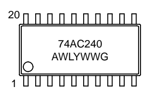
SOEIAJ-20
