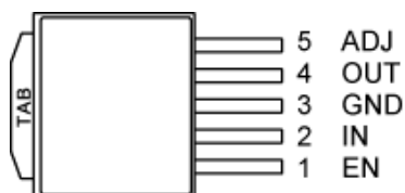
5-Pin TO-252 (D-Pak) Adjustable Voltage (D) MIC29152
