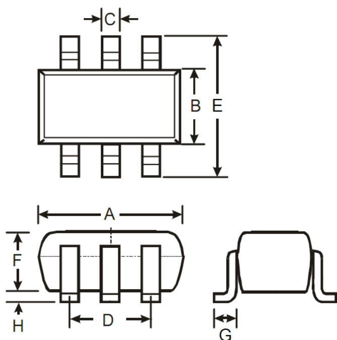
SOT-363
