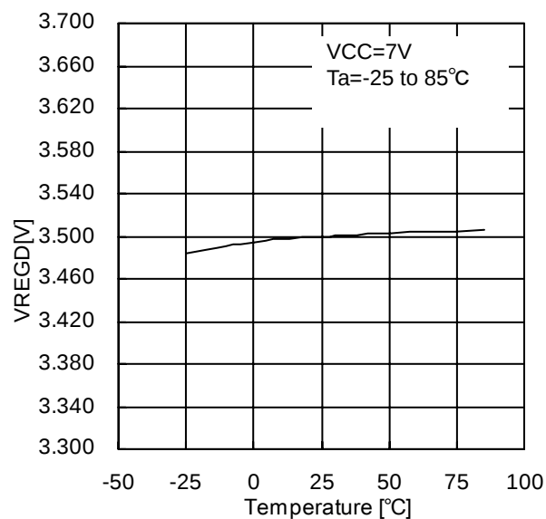
Figure.17 VREGD – Ta
