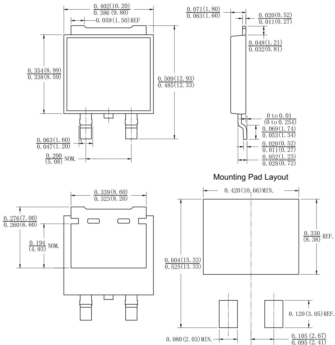
TO-263AC (SMPD)
