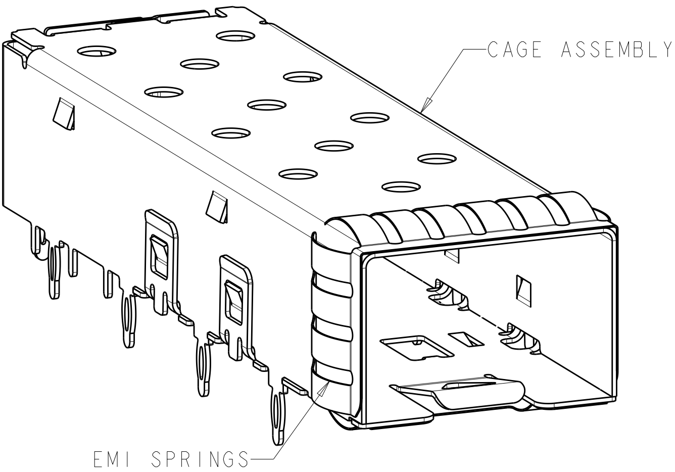
2007215-1 SCALE 5:1
