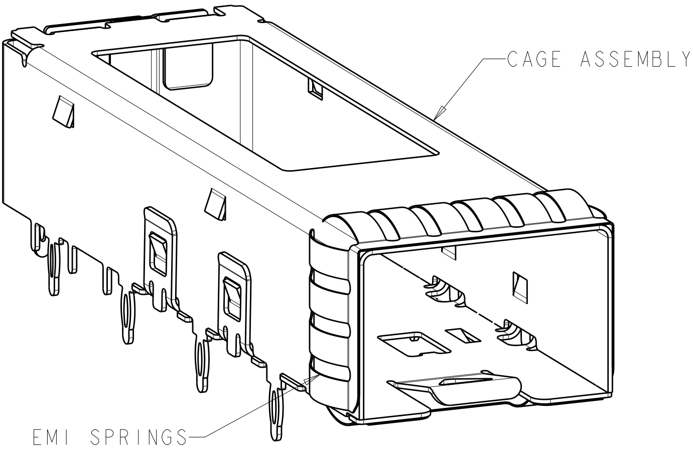
2007215-2 SCALE 5:1
