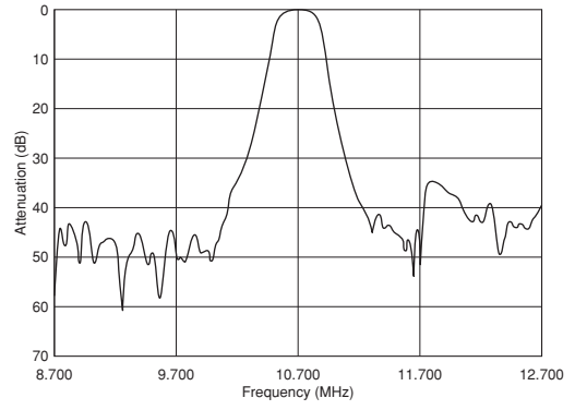
SFECF10M7EA00-R0
