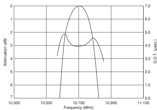
SFECF10M7HA00-R0/SFECF10M7HF00-R0
