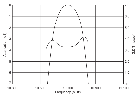
SFECF10M7GA00-R0/SFECF10M7GF00-R0
