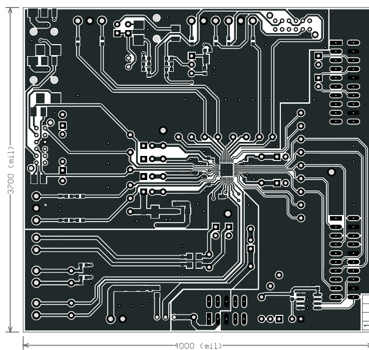
Figure C-2. Top Layer
