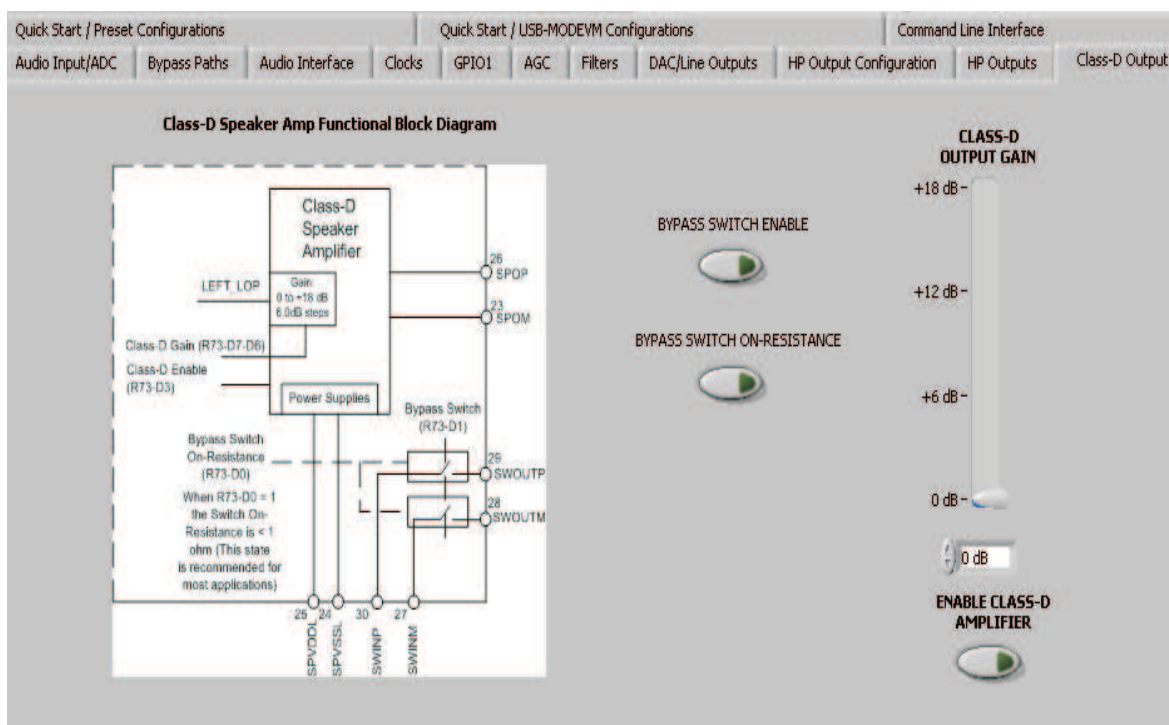
Figure 29. Class-D Output Tab
