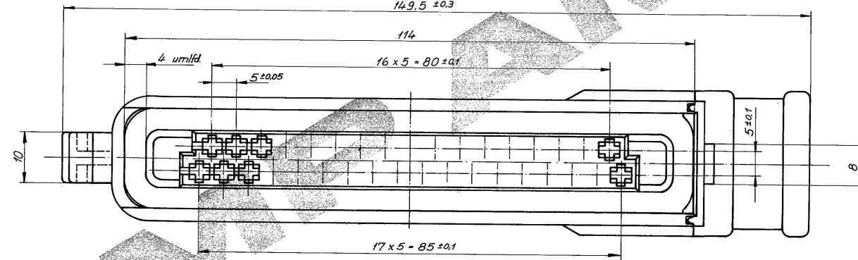
Ansicht „Y“
