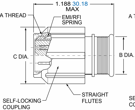
2M805-001
