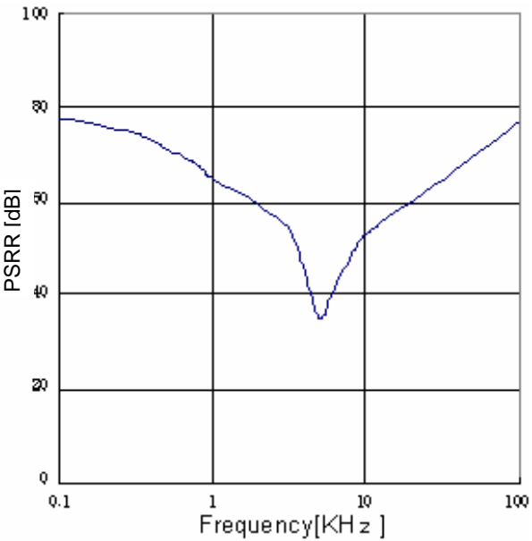
Fig.32 PSRR (Io=0mA)
