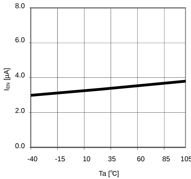
Fig.24 T_a - I_{EN}
