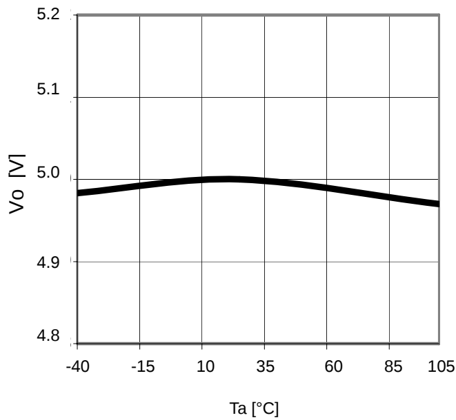
Fig.21 T_a-V_o ( I_o=0mA )
