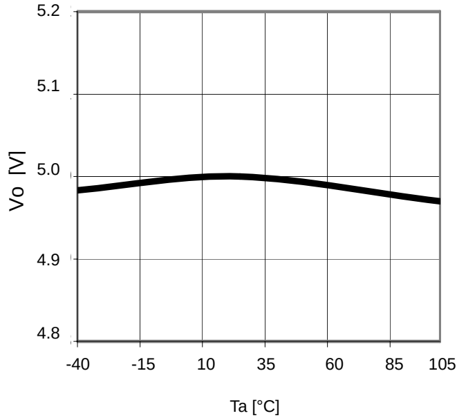
Fig.21 T_a-V_o ( I_o=0mA )
