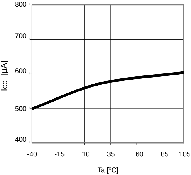
Fig.22 T_a-I_{cc}
