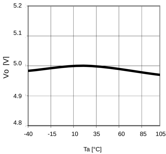
Fig.21 T_a-V_o ( I_o=0mA )
