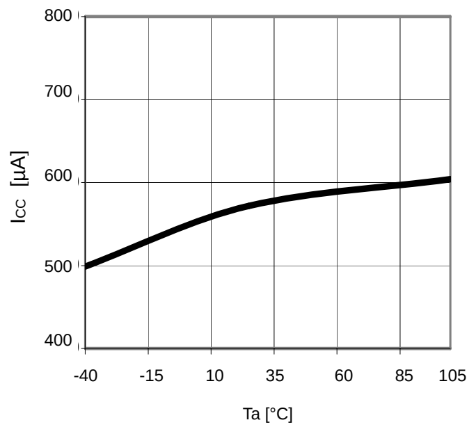
Fig.22 T_a-I_{cc}
