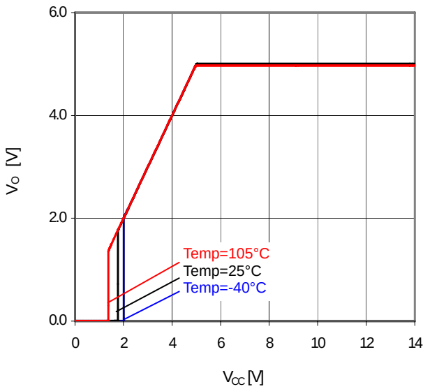
Fig.27 V_{CC}-V_o ( I_o=0mA )
