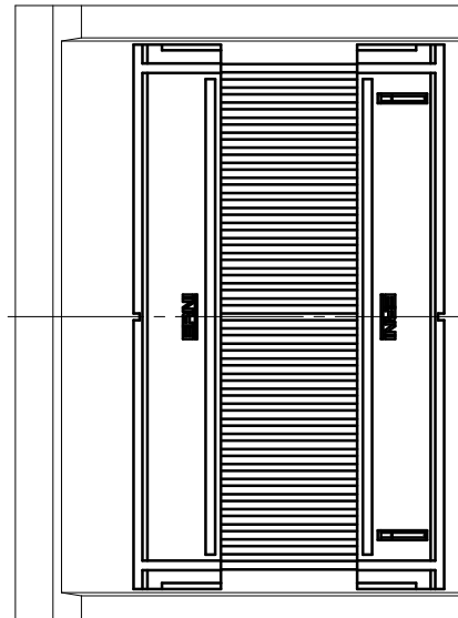
Einzelheit X (M 2:1) detail X (scale 2:1)
